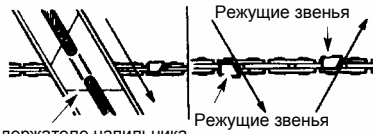
30° Отметка на держателе напильника
